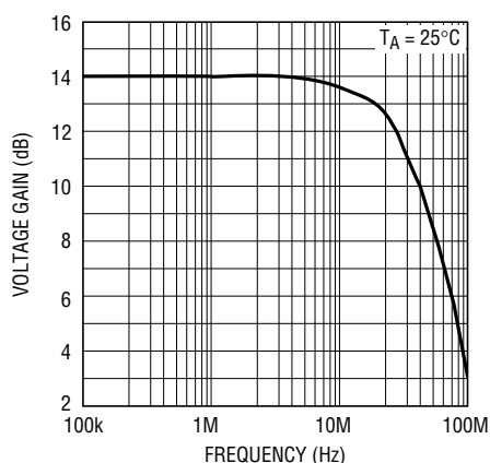
LT1194 • TA08
