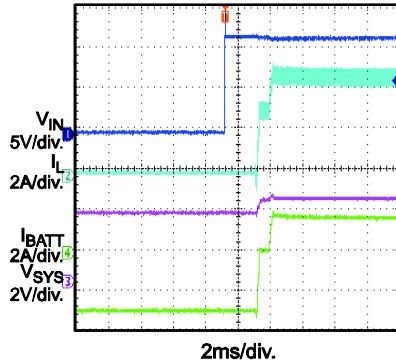
Plug in Adapter V_{BATT} = 3.7V , I_{SYS} = 3A
