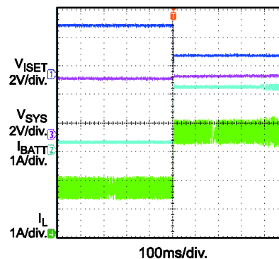
Charge On V_{BATT} = 3.7V , I_{SYS} = 1.5A
