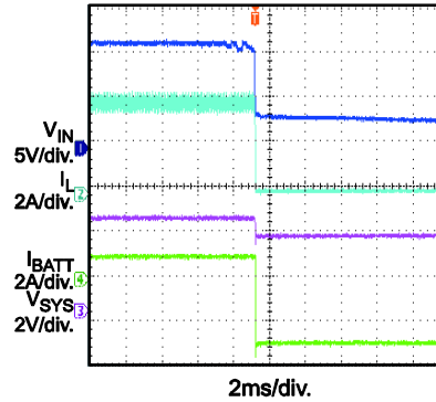
Remove Adapter V_{BATT} = 3.7V , I_{SYS} = 3A
