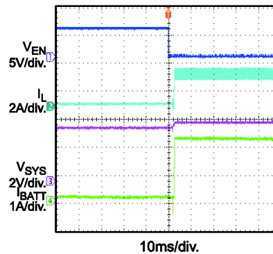
En On V_{BATT} = 3.7V , I_{SYS} = 0A
