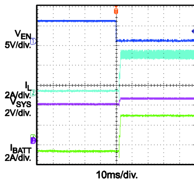
En On V_{BATT} = 3.7V , I_{SYS} = 1.5A
