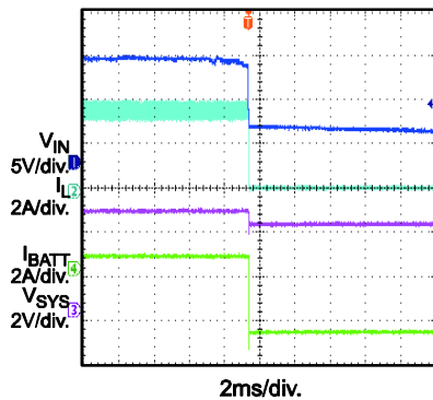
Remove Adapter V_{BATT} = 4.2V , I_{SYS} = 3A
