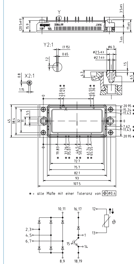
EconoBRIDGE™ Rectifier 2
