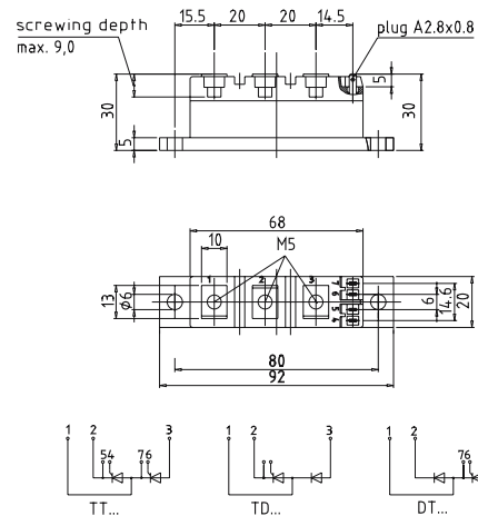
20 mm TP20
