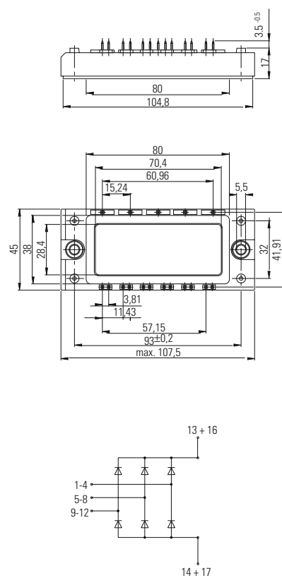
EconoBRIDGE™ Rectifier 2
