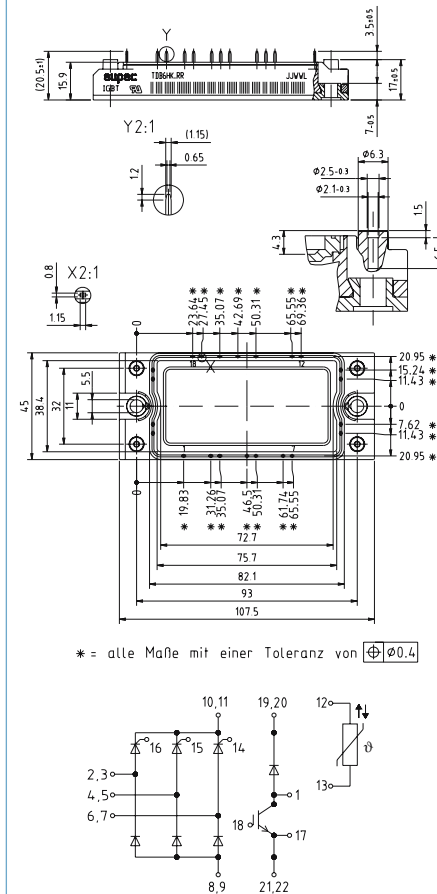
EconoBRIDGE™ Rectifier 2
