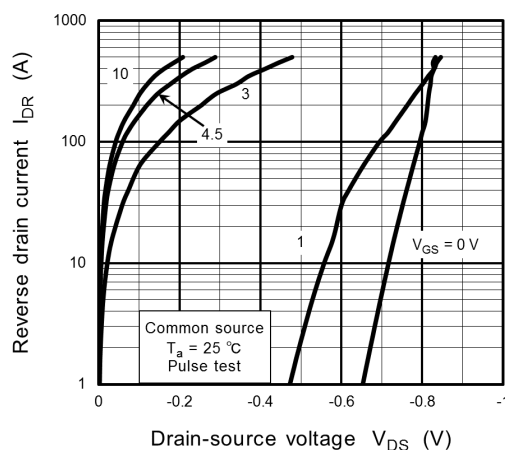
Fig. 8.6 I_{DR} - V_{DS}
