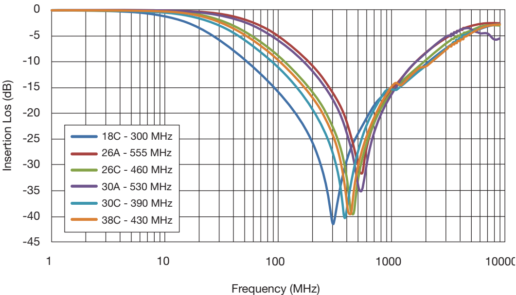
0805 Case Size
