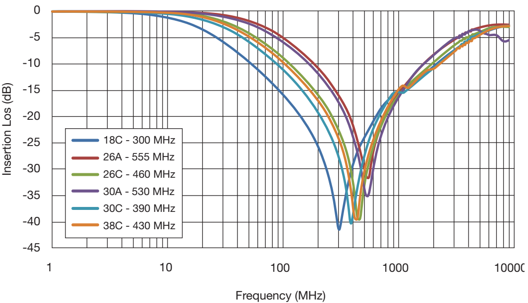
0805 Case Size
