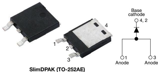
SlimDPAK (TO-252AE)
