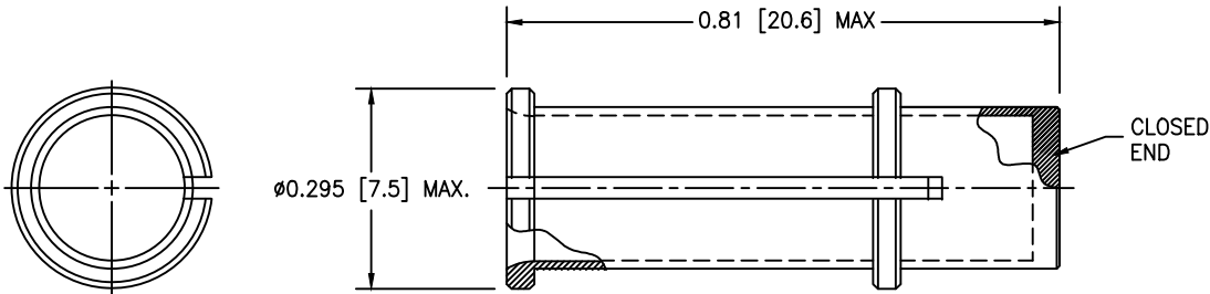
-02: PLUG
