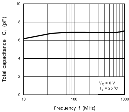
Fig. 9.4 C_t - f
