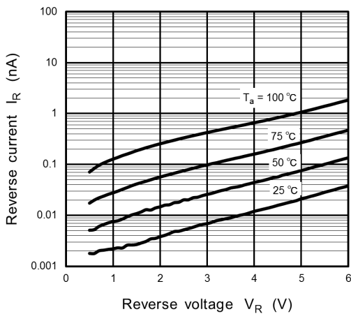
Fig. 9.2 I_R - V_R
