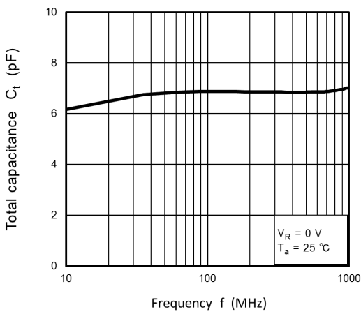
Fig. 9.4 C_t - f
