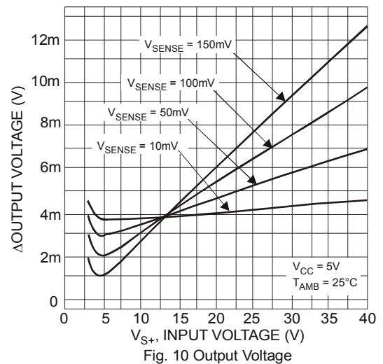
Fig. 10 Output Voltage
