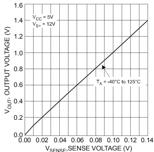
Fig. 5 Output Voltage
