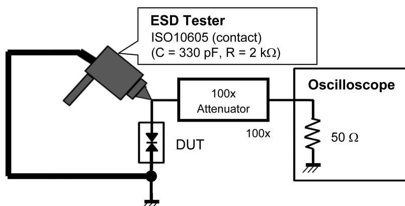
Fig. 11.5 ISO10605-4-2 (contact)
