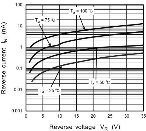
Fig. 8.2 I_R - V_R
