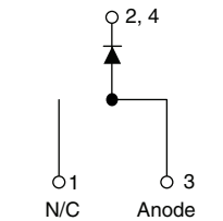
VS-ETU1506-1HM3
