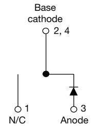
VS-ETU1506SHM3
