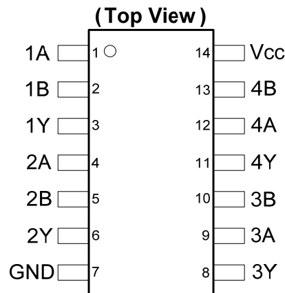
SO-14 / TSSOP-14
