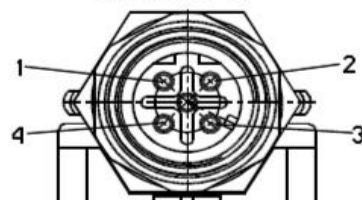
Ansicht X
