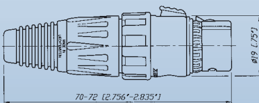
NC3MXCC
