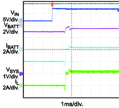
Plug in Adapter V_{BATT} = 3.7V , I_{SYS} = 2A
