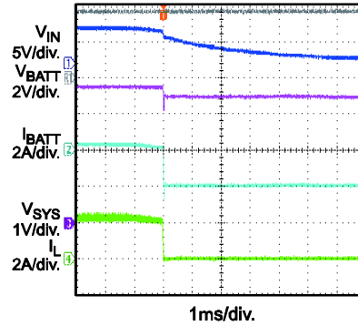
Remove Adapter V_{BATT} = 3.7V , I_{SYS} = 2A
