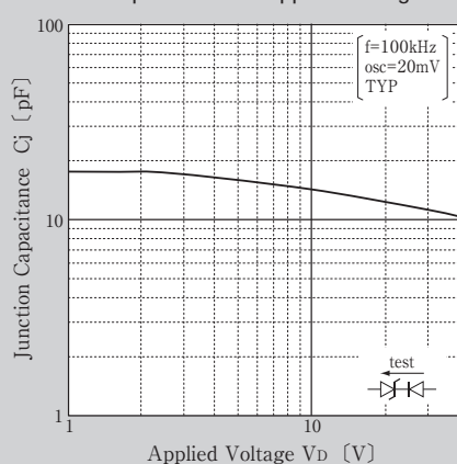
接合容量 - 印加電圧 Junction Capacitance vs Applied Voltage
