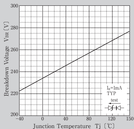
ブレークダウン電圧-接合部温度 Breakdown Voltage vs Junction Temperature
