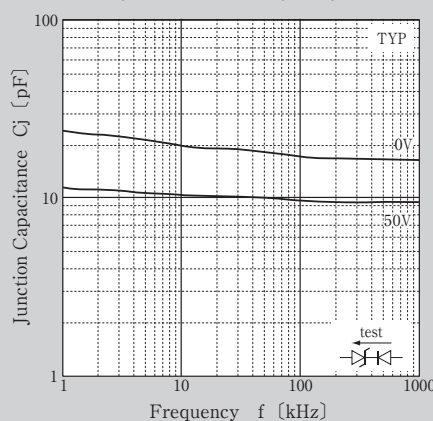
接合容量 - 周波数 Junction Capacitance vs Frequency
