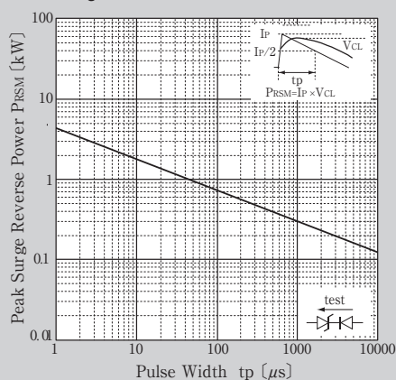
せん頭サージ逆電力 Peak Surge Reverse Power
