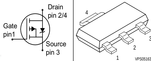
PG-SOT223
