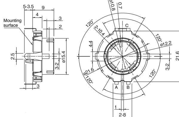
EC21A Actuator length 9mm 9 pulse/18 detent
