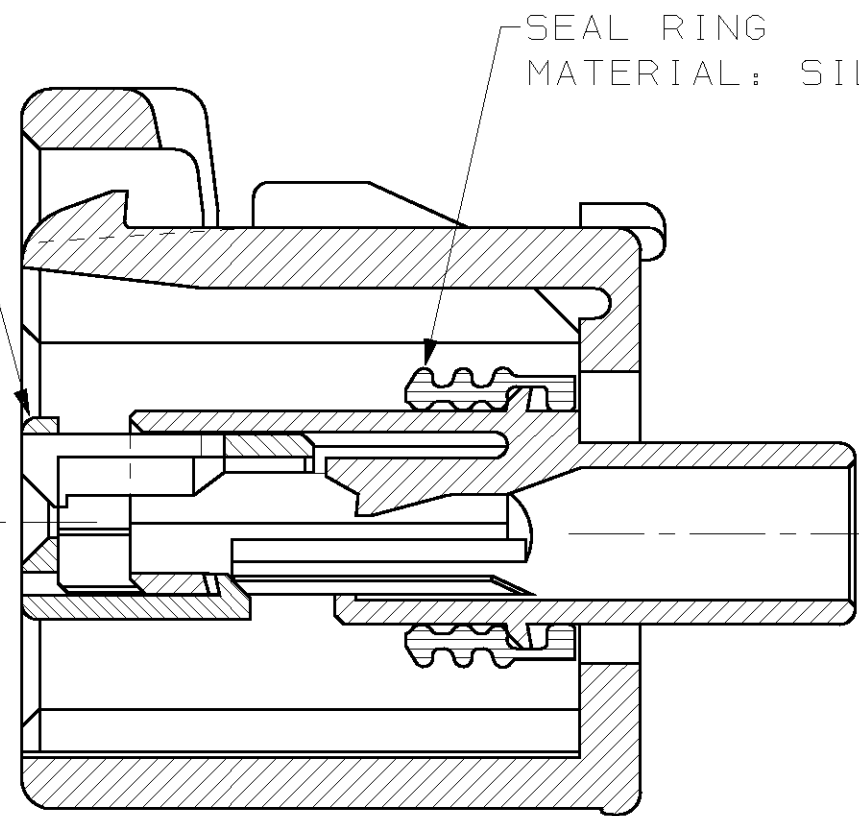
SECTION A-A
