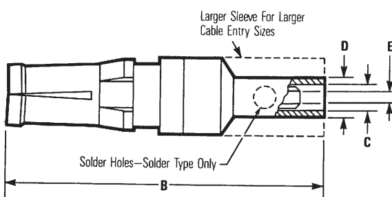
Receptacle
