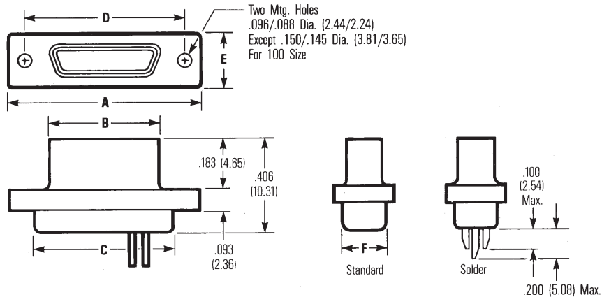
Socket
