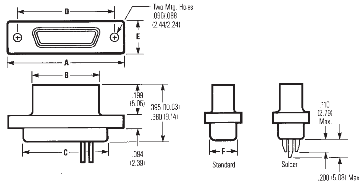
Socket
