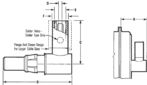
Receptacle
