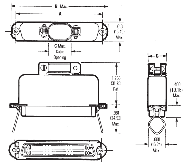
Socket
