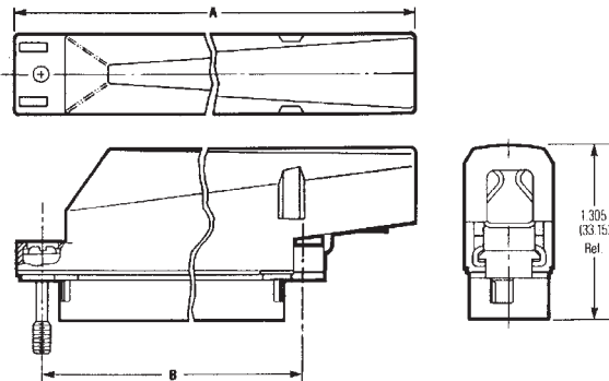
Socket
