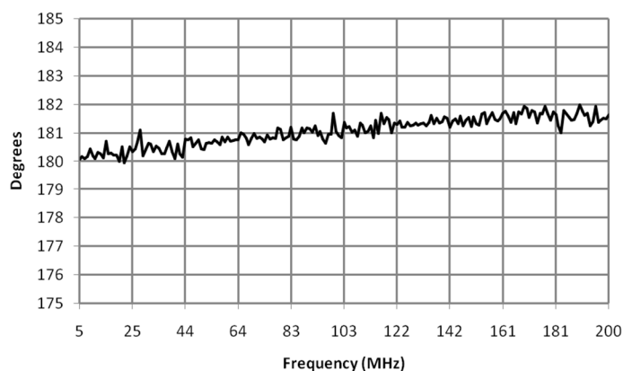
MABA-011048 phase_balance
