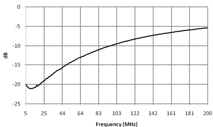
MABA-011048 input_return_loss_pin6
