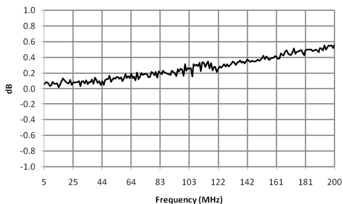
MABA-011048 amplitude_balance
