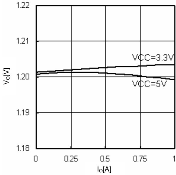
Fig.15 Io-Vo (Vo=1.2V)
