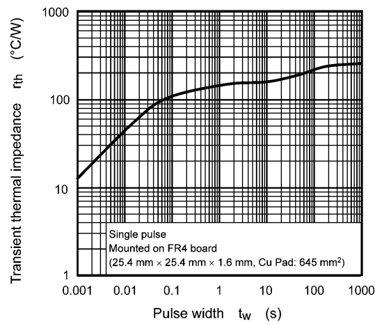
Fig. 8.13 r_{th} - t_w
