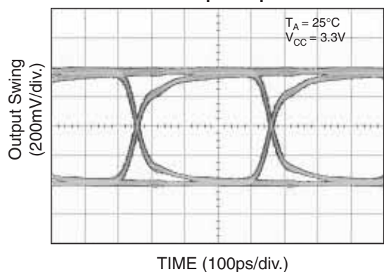
2.5Gbps Output
