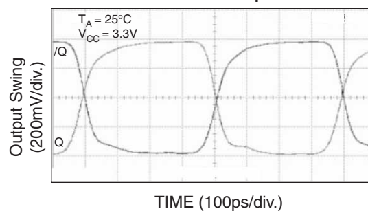
1.25GHz Output
