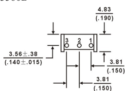
TSR-3386C
