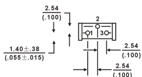
TSR-3386J
