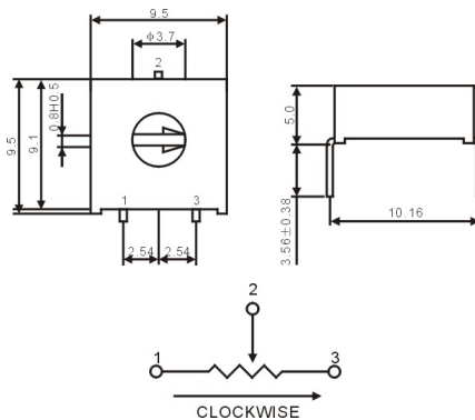
TSR-3386G
