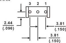
TSR-3386S
