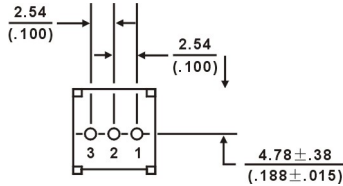
TSR-3386Y
