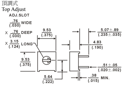
TSR-3386F
