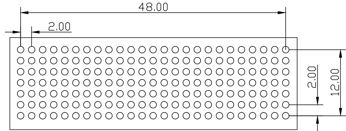
LAY-OUT P.C.B.-HOLE
