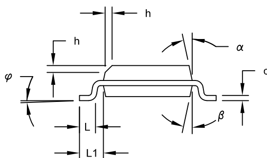
VIEW A-A
