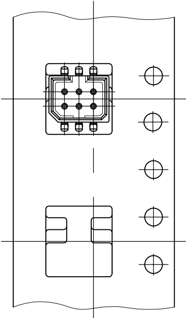
6 Pos. (P/N: 3-176890-6)
