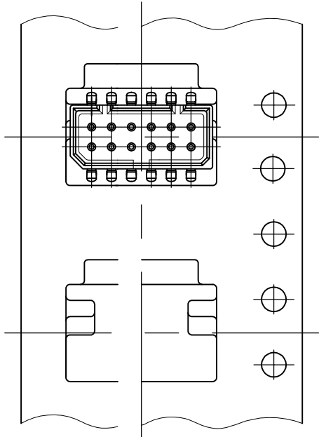
12 Pos. (P/N: 7-176890-2)
