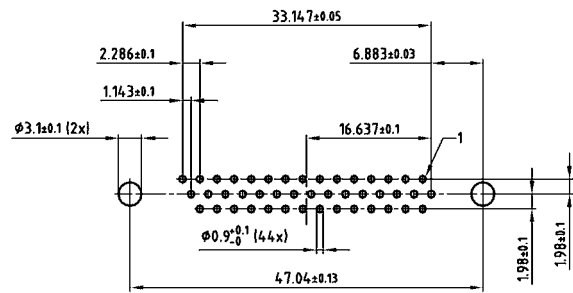
44 POS.
