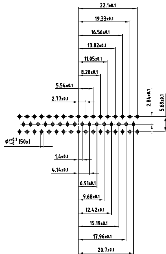
50 pos.
