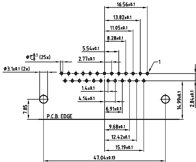
25 POS.
