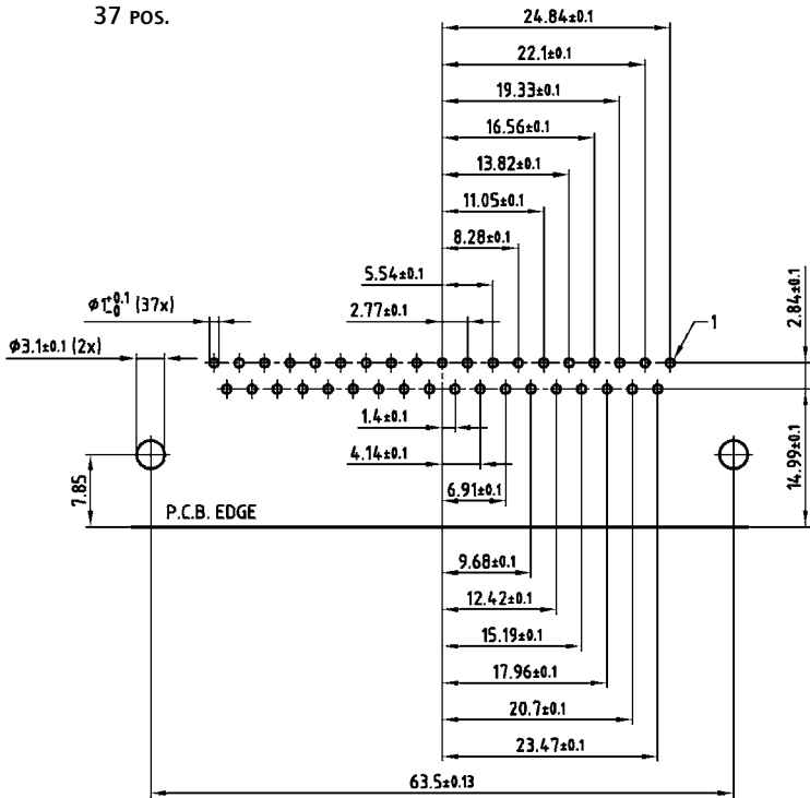
37 POS.
