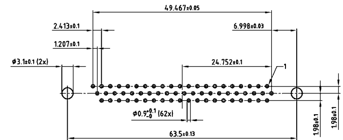
62 POS.
