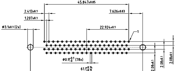
78 POS.
