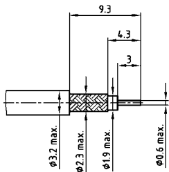
verwendbare Kabel: RG- 174U, 188AU, 316U Usable Cables
