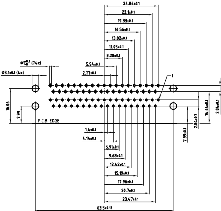
2x37 POS.
