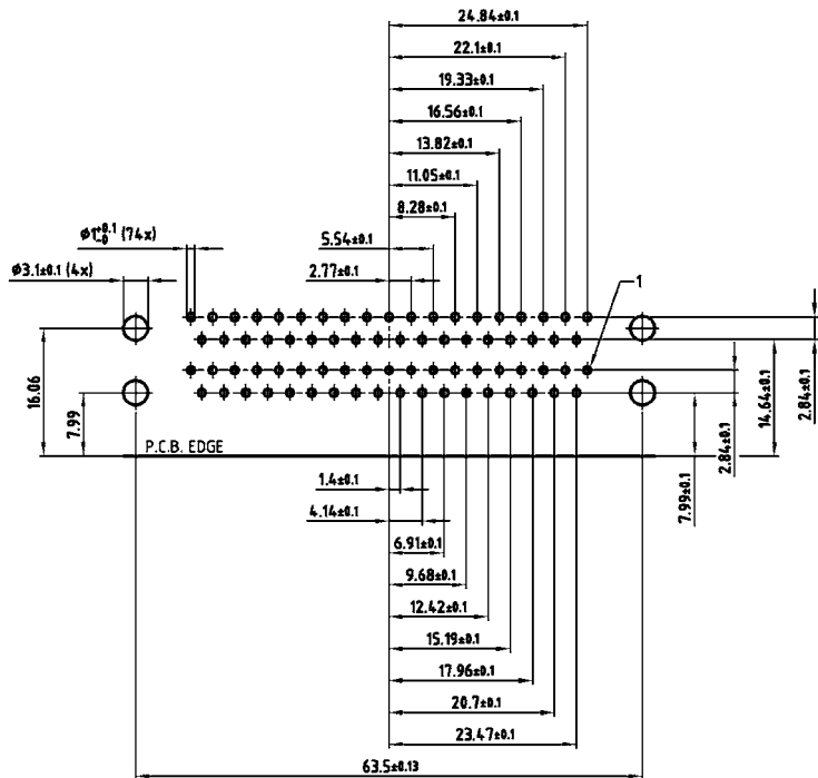
2x37 POS.
