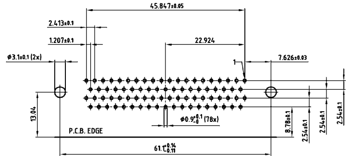
78 POS.
