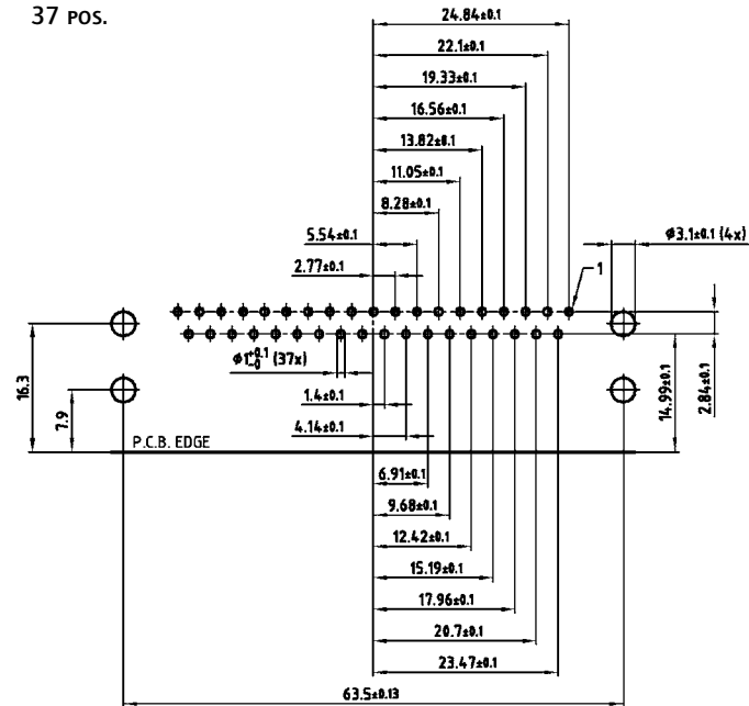
37 pos.
