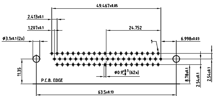
62 POS.
