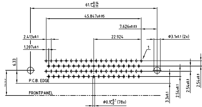
78 pos.
