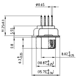
78 pos. = Dim. in ( _ )
