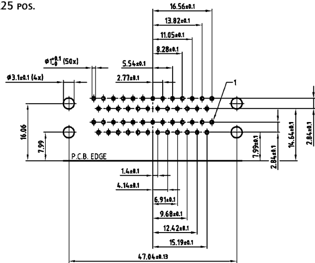
2x25 POS.
