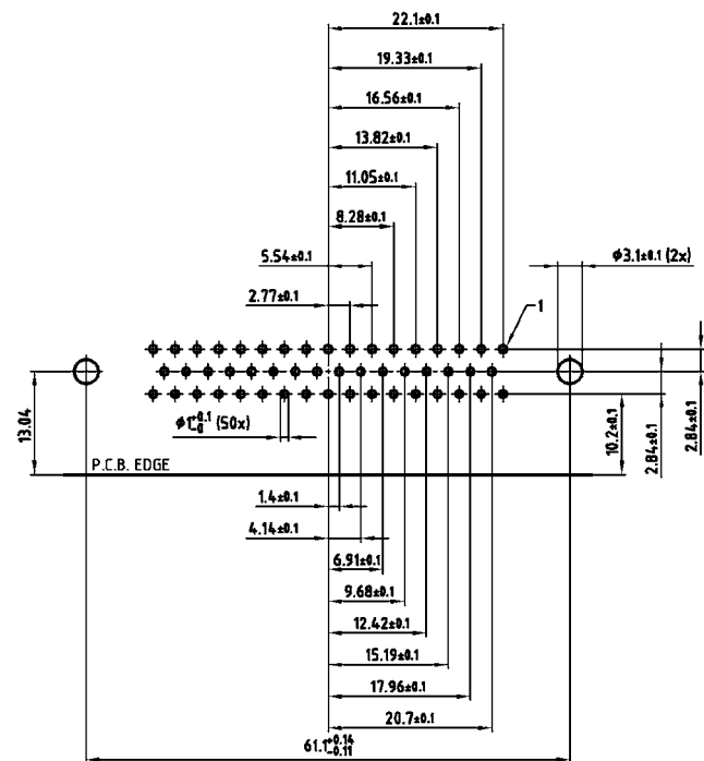
50 pos.
