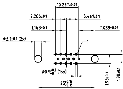
15 POS.
