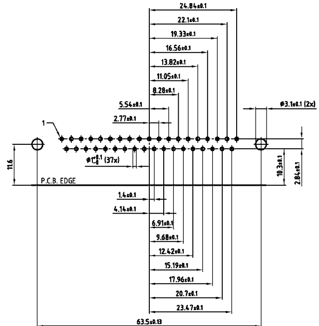
37 POS.
