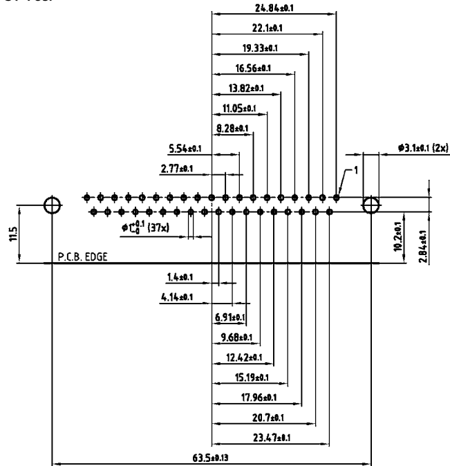
37 POS.
