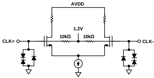
Figure 26. CLK± Inputs
