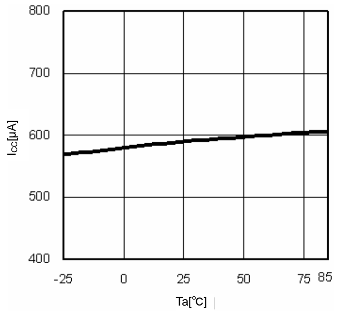
Fig.9 T_a-I_{CC}
