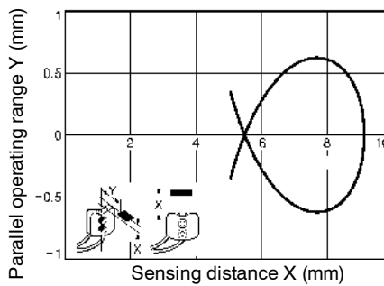
E32-L25L with E3X-DAN amplifier
