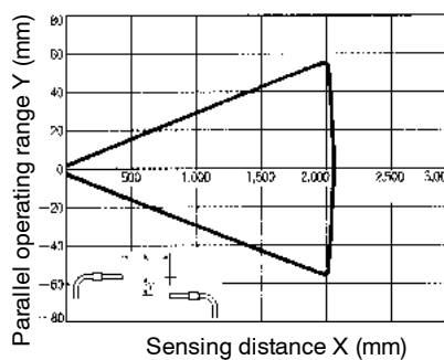
E32-T84S with E3X-NH amplifier
