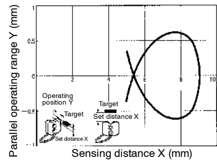
E32-L25L with E3X-NH amplifier
