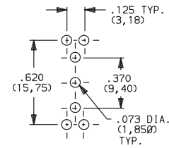
E101J1_BE2 SPDT
