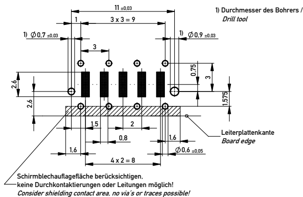
Leiterplatten-Layout Vorschlag / PCB-layout proposal
