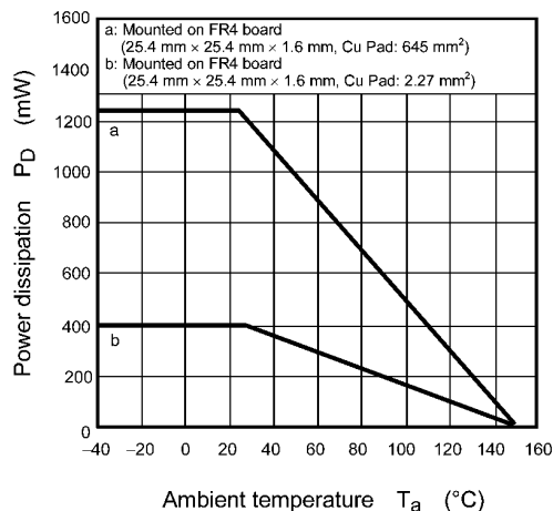
Fig. 7.14 P_D - T_a
