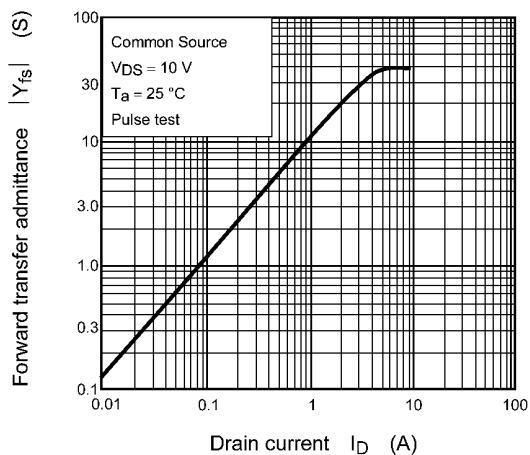
Fig. 7.8 |Y_{fs}| - I_D
