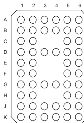
52-Ball BGA
