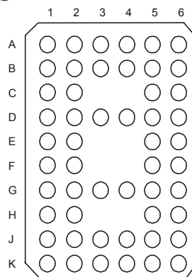
52-Ball BGA
