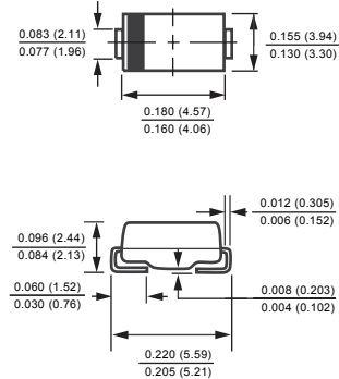
DO-214AA
