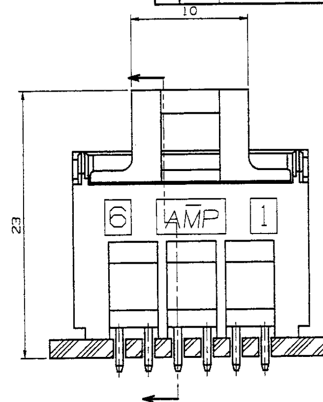
ダストカバー取付状態図
