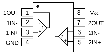
SO-8/TSSOP-8/MSOP-8
