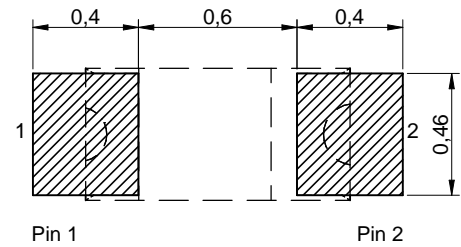
Scale - 35:1
