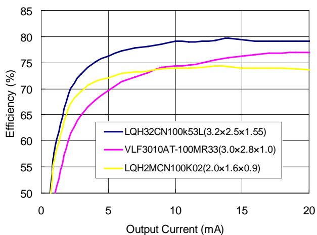
V_{OUT}=20V, V_{IN}=3.6V
