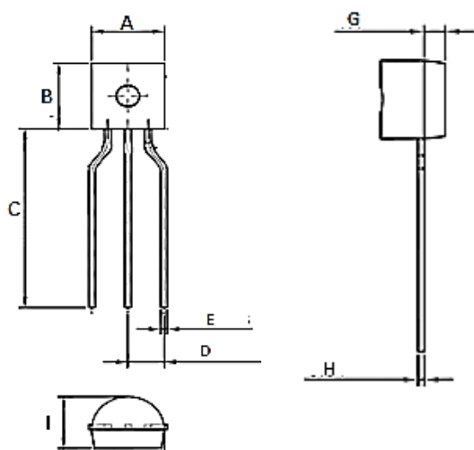
TO-92 Ammo
