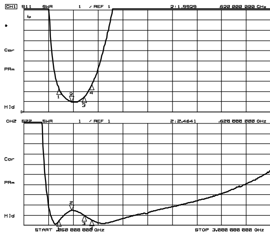
VSWRi, VSWRo
